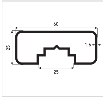
0,658 kg/m ER.8226
