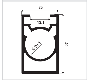
0,774 kg/m ER.8231
