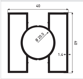
0,900 kg/m ER.8229
