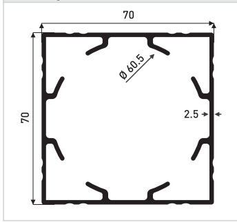
2,422 kg/m ER.8232
