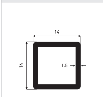
0,201 kg/m ER.8236
