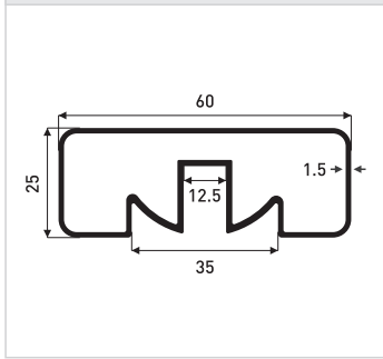
0,865 kg/m ER.8224
