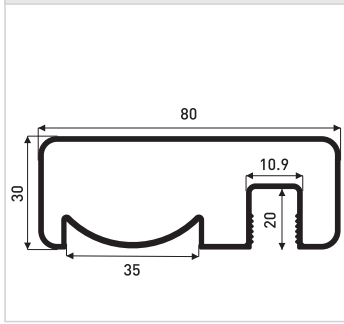
1,110 kg/m ER.8220
