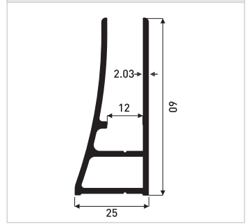
0,892 kg/m ER.8235
