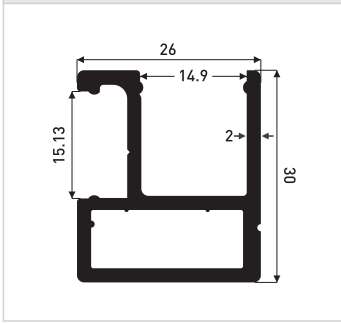
0,620 kg/m ER.8233
