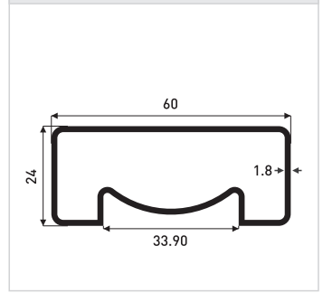
0,837 kg/m ER.8223
