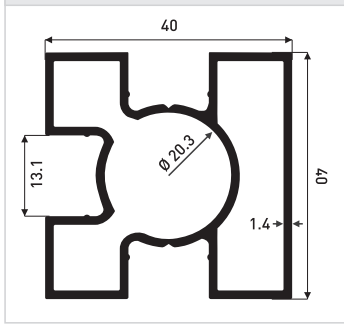
0,890 kg/m ER.8228
