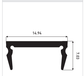
0,088 kg/m ER.8239
