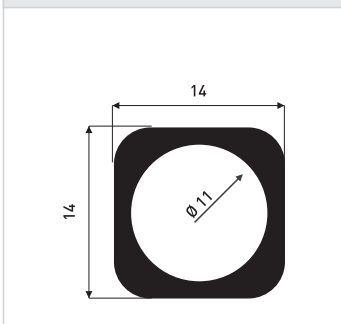
0,251 kg/m ER.8237
