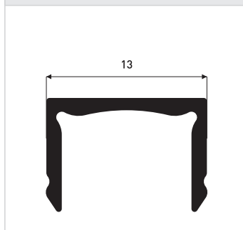
0,090 kg/m ER.8238
