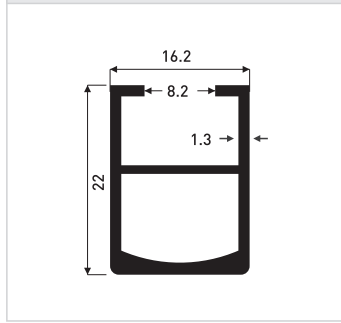
0,286 kg/m ER.8234
