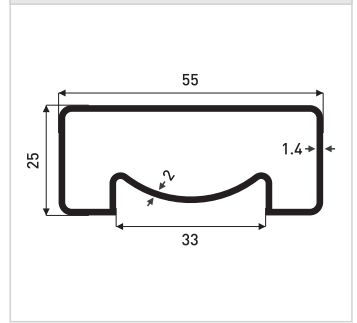
0,658 kg/m ER.8227
