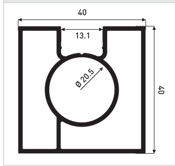
0,895 kg/m ER.8230
