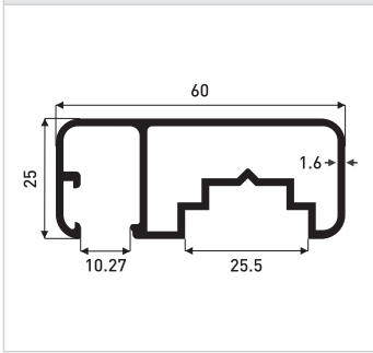
0,864 kg/m ER.8225
